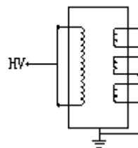
图 6-2 P1 接法
