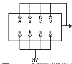
图 6-10 文/压器反接法
