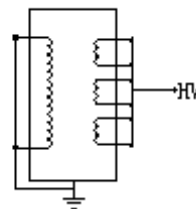
图 6-3 PT 接法
