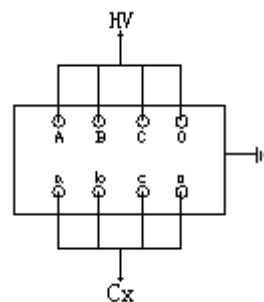
图 6-9 文/压器接法
