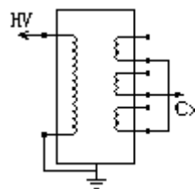
图 6-4 PT 末屏法
